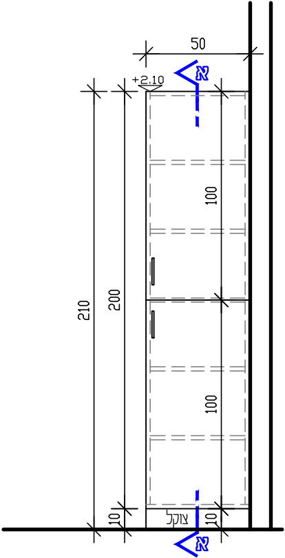
חזית קנ"מ 25'
