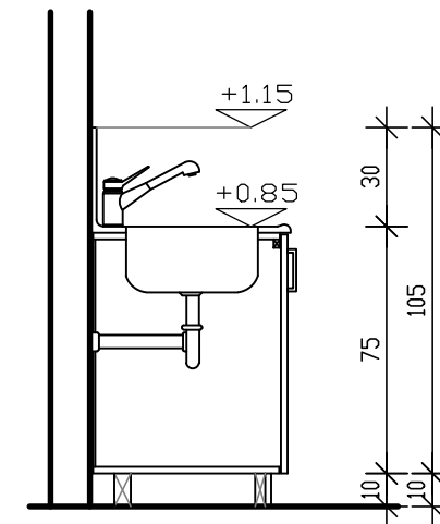
חתך א-א קנ"ח 1:25
