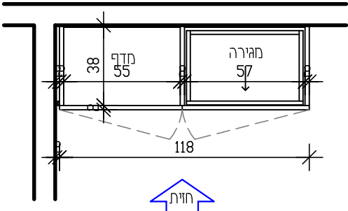
תוכנית מתחת המשטח קנ"מ 25:1
