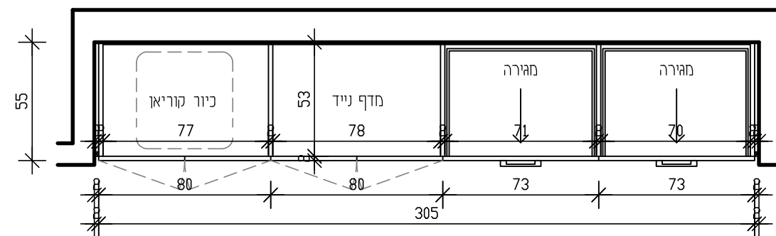
תוכנית מתחת המשטח קנ"מ 25:
