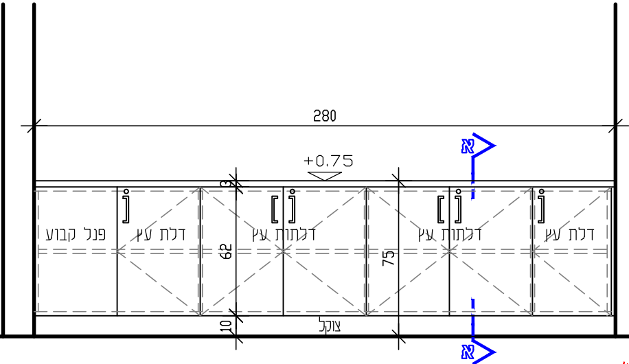
תוכנית מתחת המשטח קנ"מ 25:1
