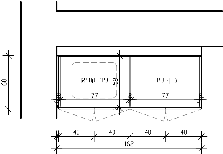
תוכנית מתחת המשטח קנ"מ 25
