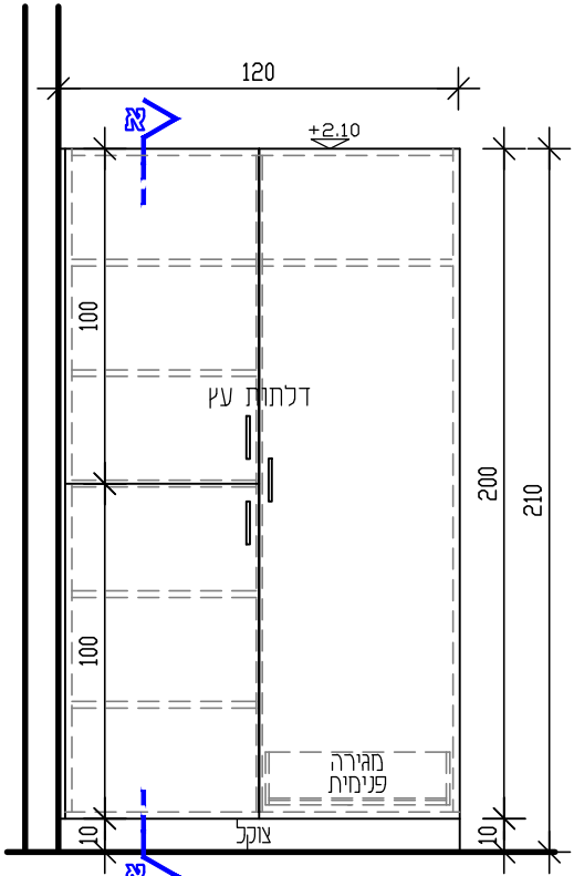
חזית קנ"מ 25:1
