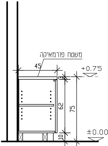
חתך א-א קנ"מ 1:25
