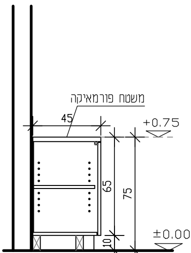
חתך א-א ארון קנ"מ 25:1
