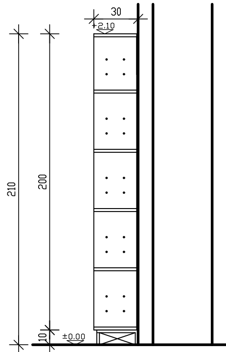
חתך א-א קנ"מ 25:1
