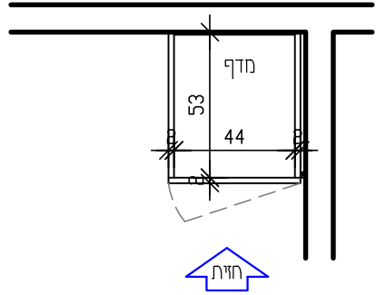
תוכנית מתחת המשטח קנ"מ 25'
