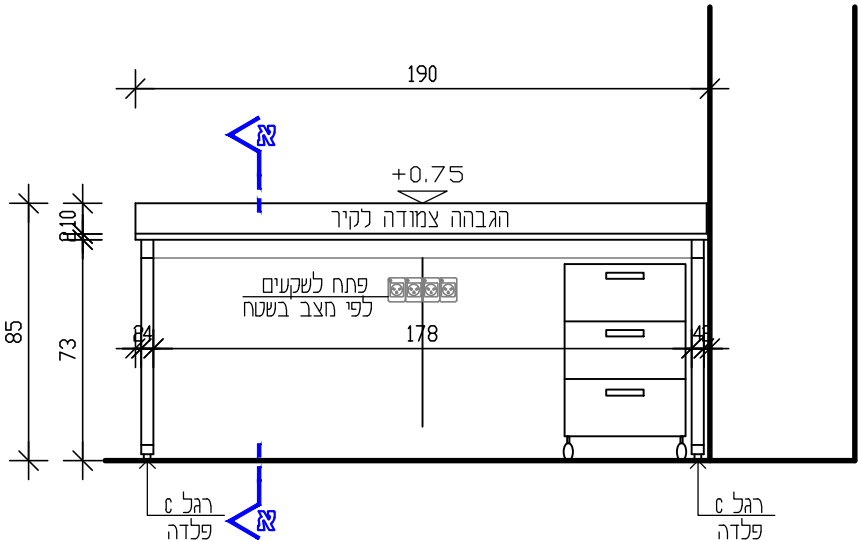
חזית המשטח קנ"מ 25:
