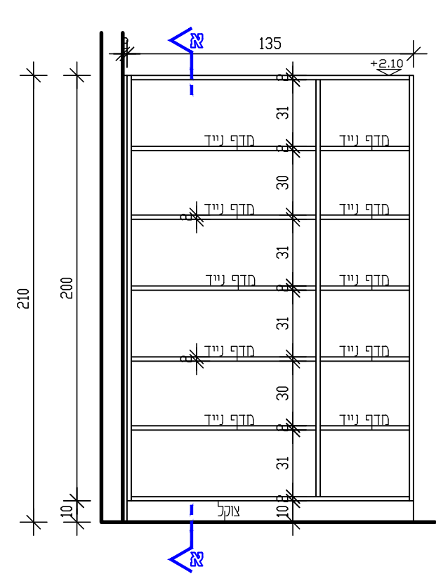
חזית פנימית קנ"מ 25:1
