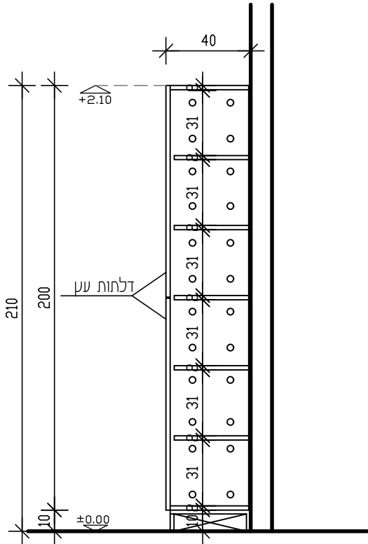
חתך A-A קנ"מ 25:1
