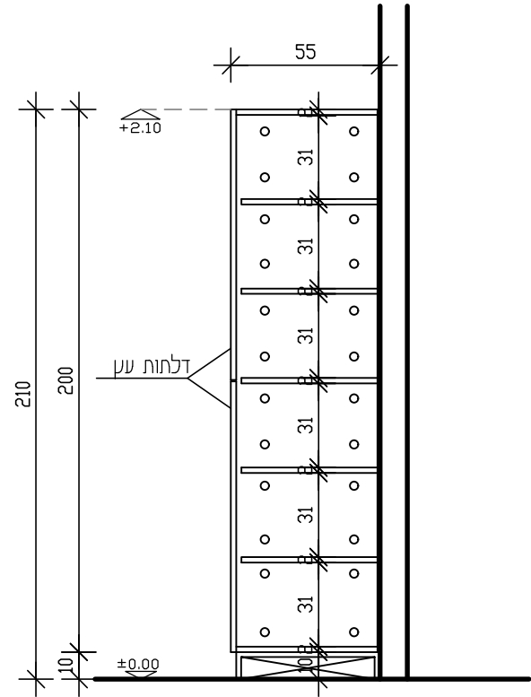
חתך א-א קנ"מ 25'
