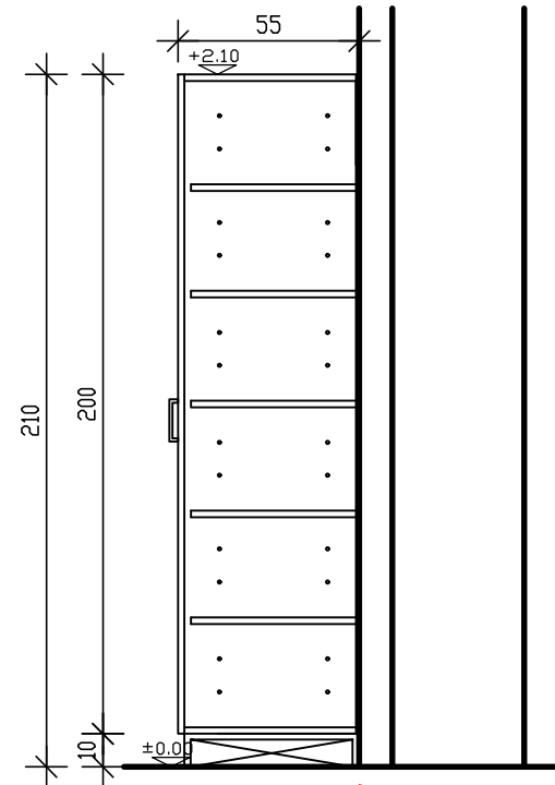
חתך א-א קנ"מ 25:1
