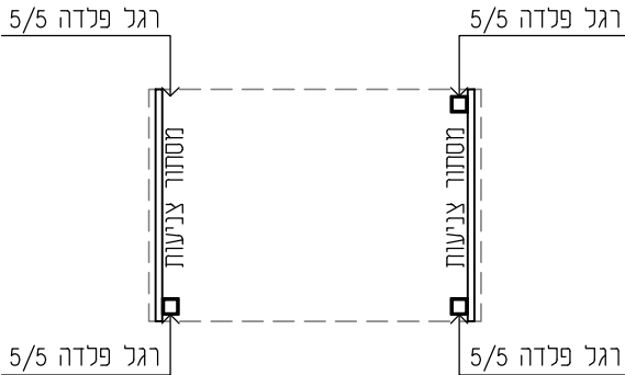
תוכנית מעל המשטח קני'מ 1:25
