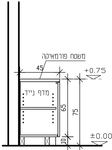
חתך א-א קנ"מ 25:1
