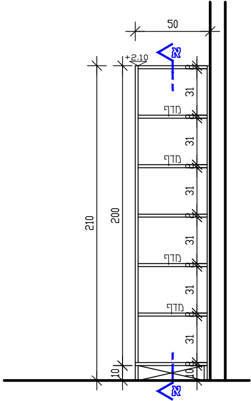
חזית פנימית קנ"מ 25'
