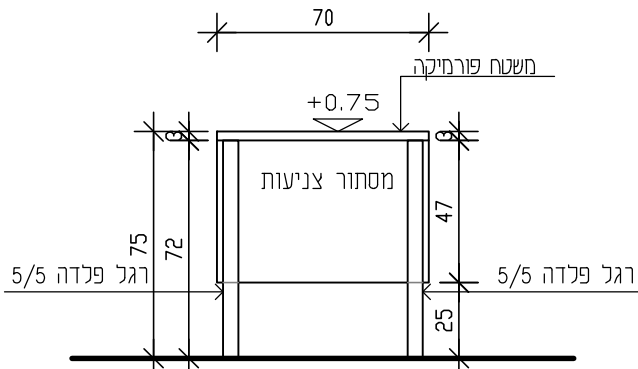
חתך א-א שולחן קני'מ 1:25
