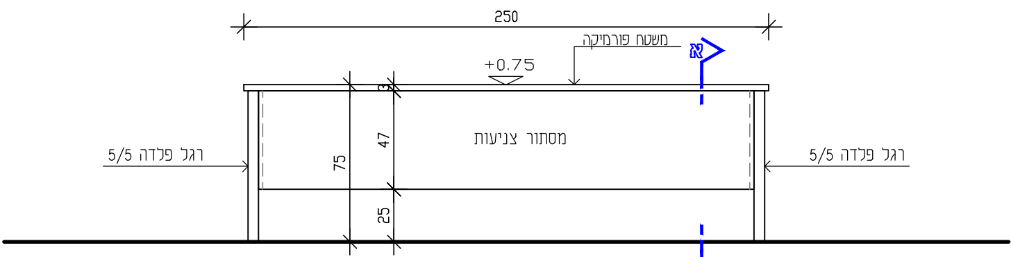
חזית שולחן קנ"מ 25:1
