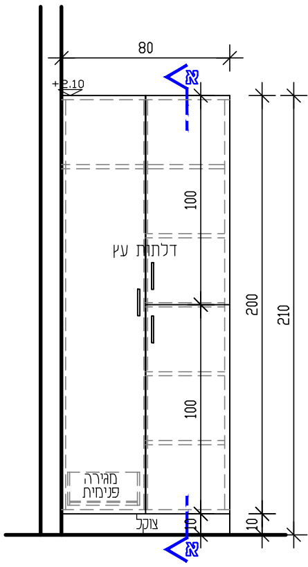
חזית קנ"מ 25
