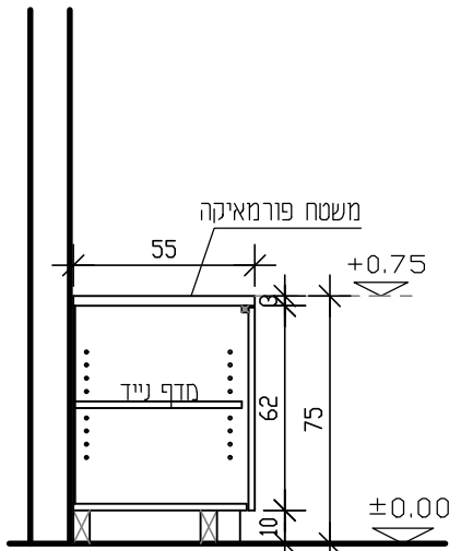
חתך א-א קנ"מ 25:1
