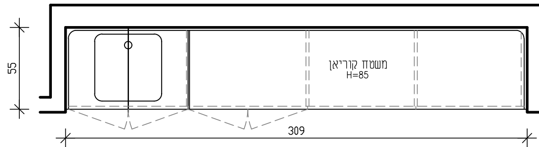
תוכנית מעל המשטח קנ"ח 25:
