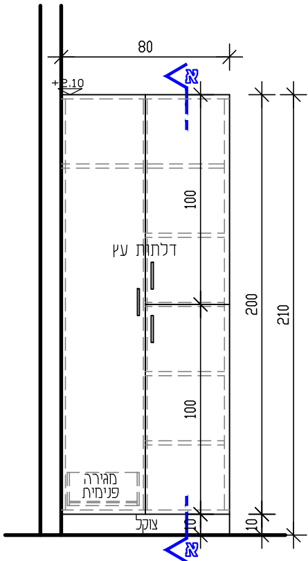
חזית קנ"מ 25
