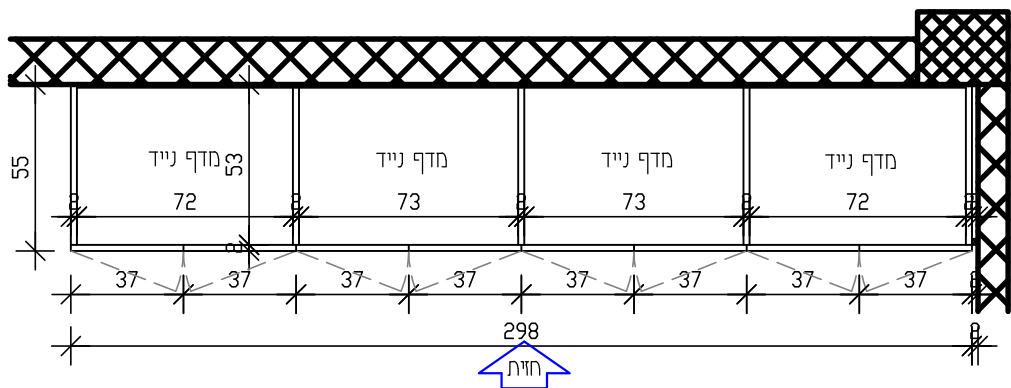
תוכנית מתחת המשטח קנ"מ 25:1
