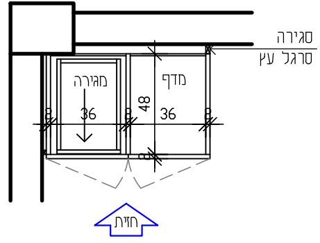
תוכנית מתחת המשטח קנ"מ 25
