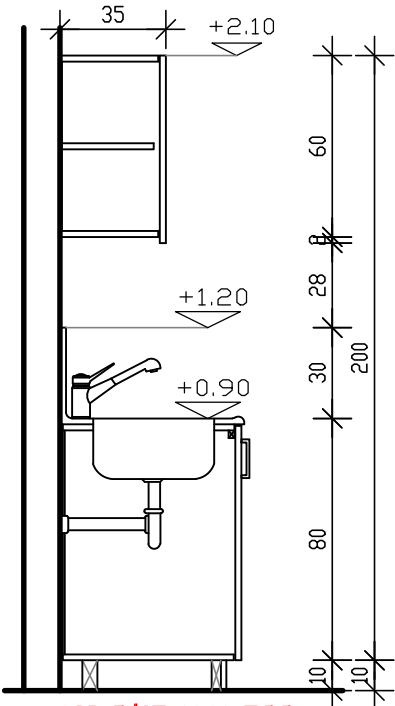
חתך א-א קנ"מ 1:25
