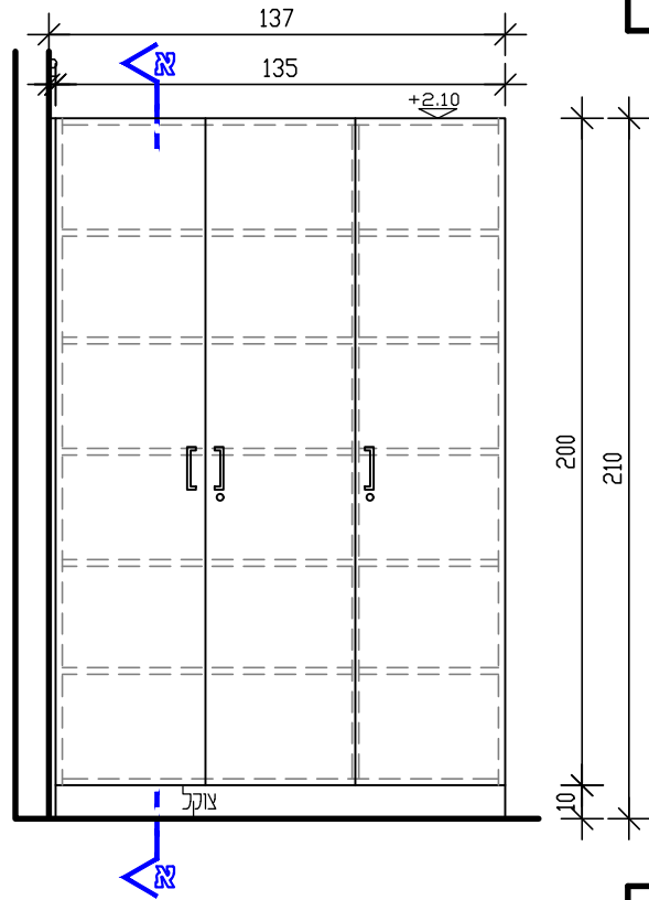
חזית חיצונית קנ"מ 25:1
