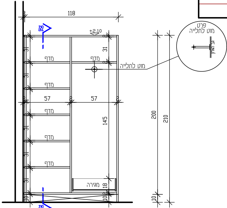
חזית פנימית קנ"מ 25:1
