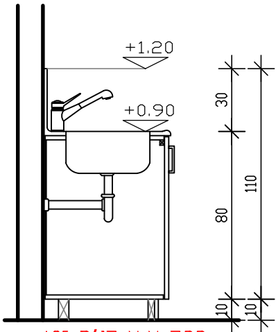
חתך א-א קנ"מ 25
