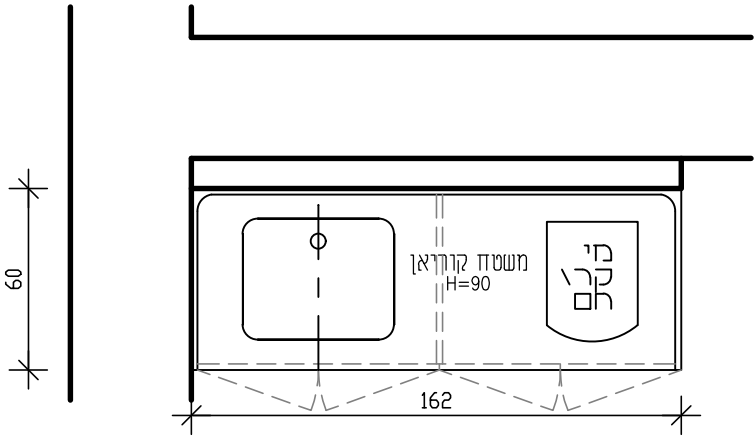
תוכנית מעל המשטח קנ"מ 25
