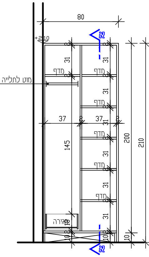
חזית פנימית קנ"מ 25
