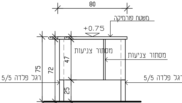
חתך א-א שולחן קנ"מ 25:1
